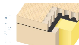
Aufbau 32mm (B1 29mm)
