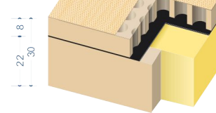
Aufbau 30mm
